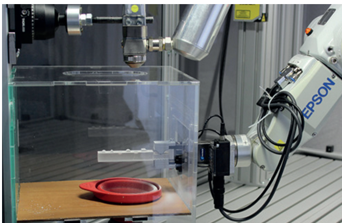
Prozessmodul zur optischen Oberflächenaufbereitung und 3D-Digitalisierung (© ITW e. V. Chemnitz)
